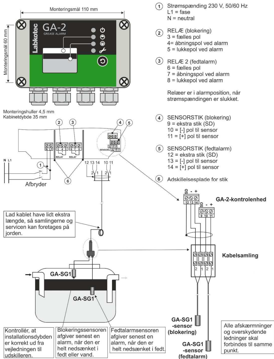
Figur 3. Installation af GA-2-fedtalarmerheden.
