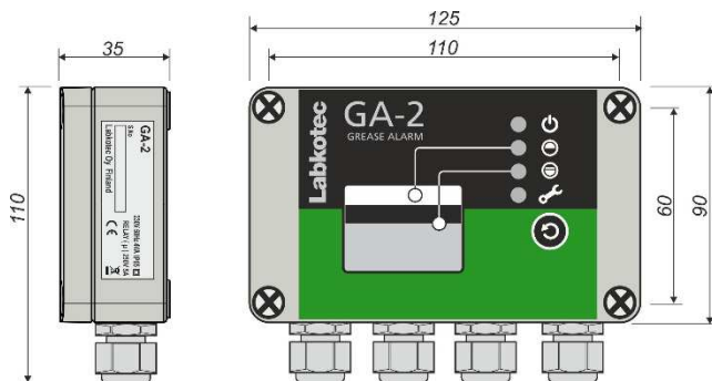
Figur 7. GA-2-kontrolenhed
