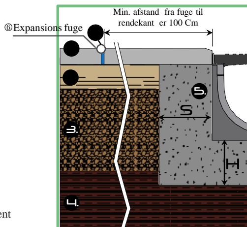
Eks. 2 Betongulv (A15-B125-C250-D400 14 )
